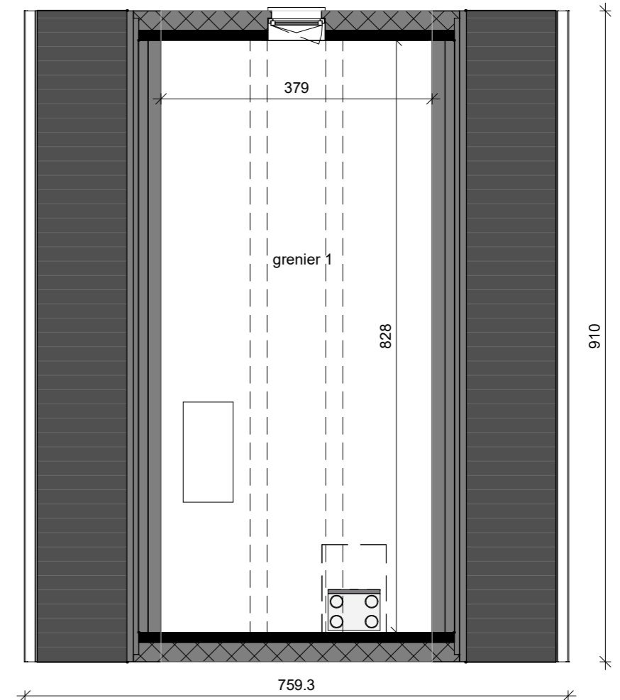
grenier surf. brute 34.49 m 2
