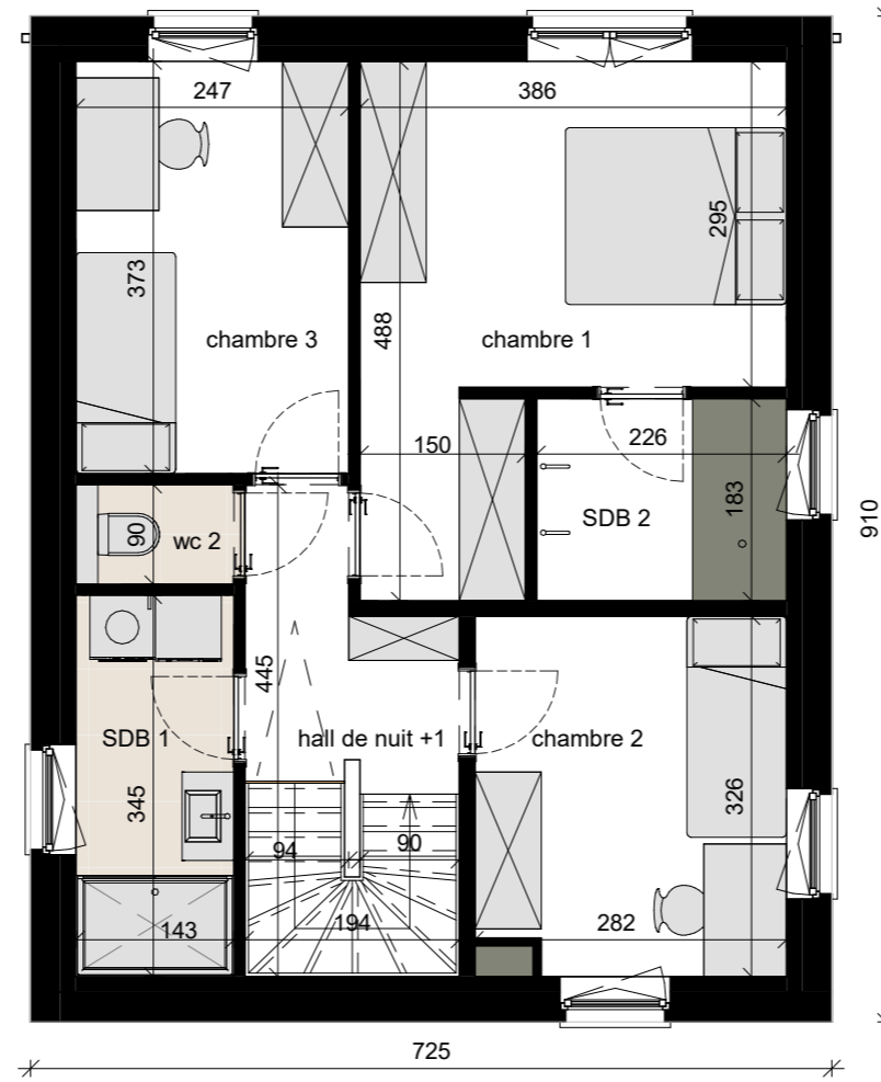
étage surf. brute 65.98 m 2
