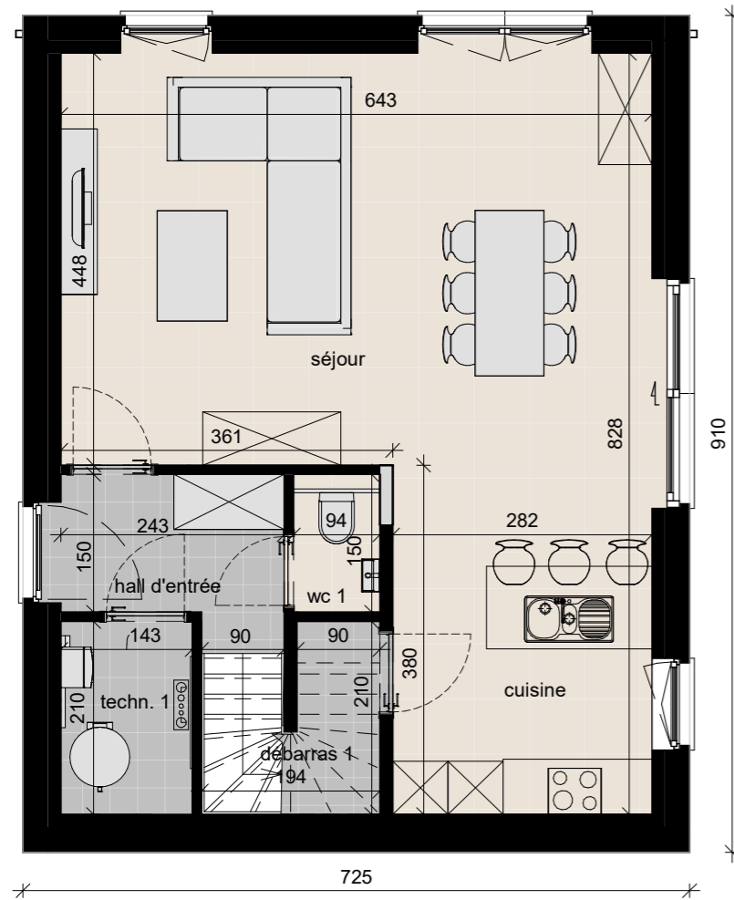
rez-de-chaussée surf. brute 65.98 m 2
